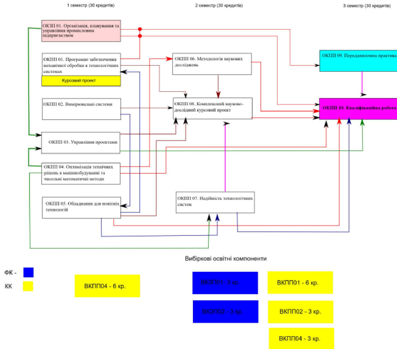
Структурно-логічна схема освітньої програми «Металорізальні верстати та системи»
